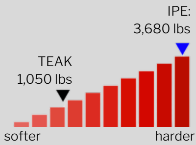
Ipe Hardness
